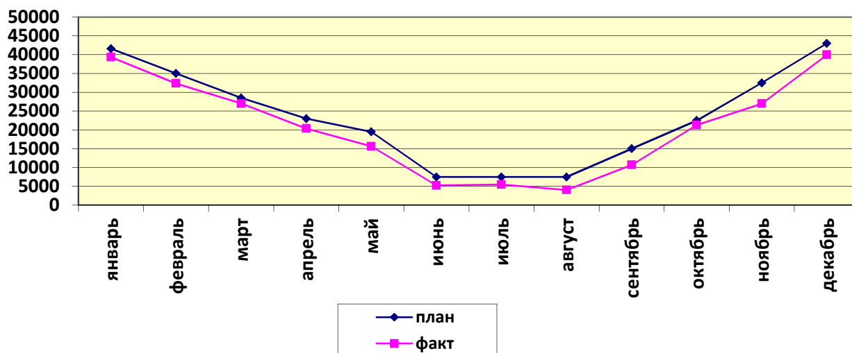
Динамика товарного отпуска электроэнергии (в тыс. кВтч)
